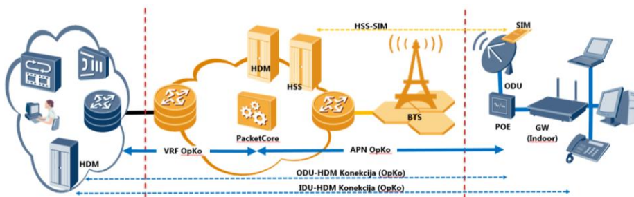
Slika 2 Shematski prikaz BSB usluge s razgraničenjem odgovornosti
