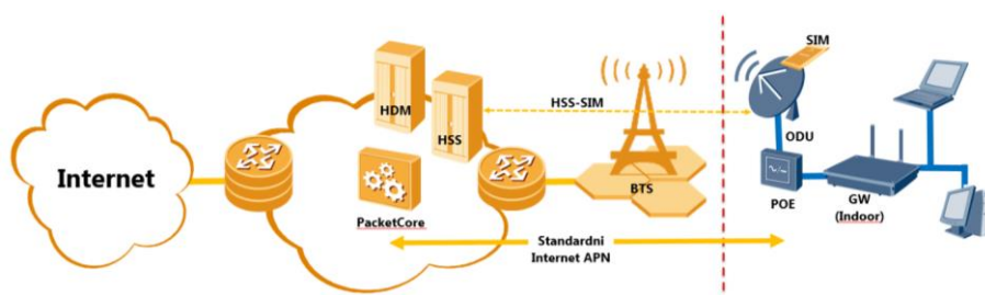
Slika 1 Shematski prikaz PB usluge s razgraničenjem odgovornosti
